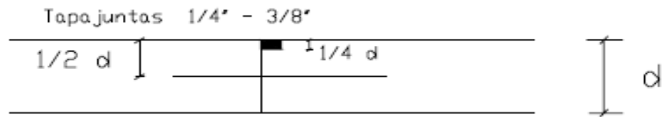
Figura 3. Transversales de contracción.
