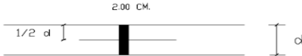
Figura 2. Junta de expansión con o sin barra de transferencia.
