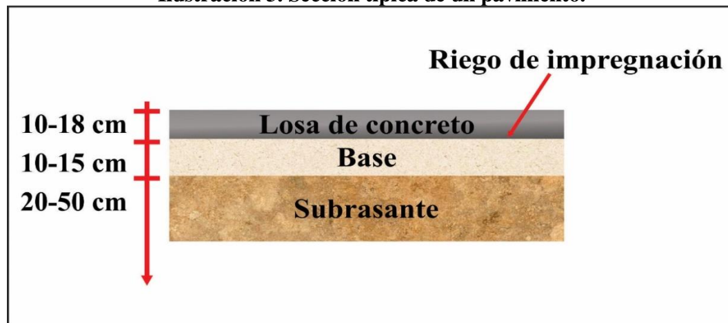
Ilustración 3. Sección típica de un pavimento.
