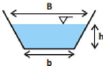
Figura No. 3 Sección de canal trapezoidal
