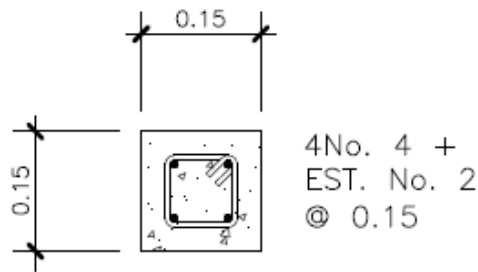
DETALLE DE COLUMNA C-1
