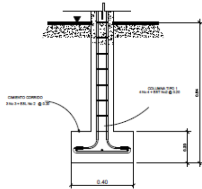
DETALLE CIMENTO CORRIDO 2
